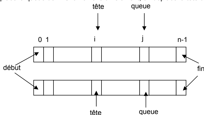
Figure XI.1 - Une file représentée en anneau continu.
