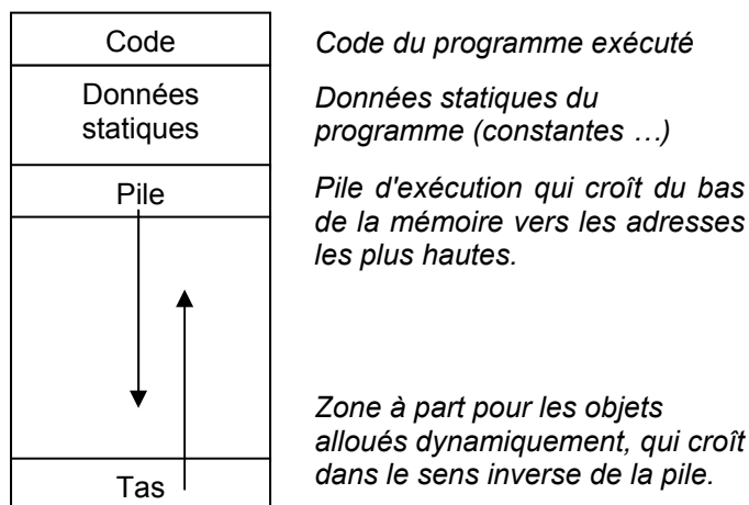
Figure X.3 - L'organisation de la mémoire d'un ordinateur à l'exécution d'un programme [AU93].
