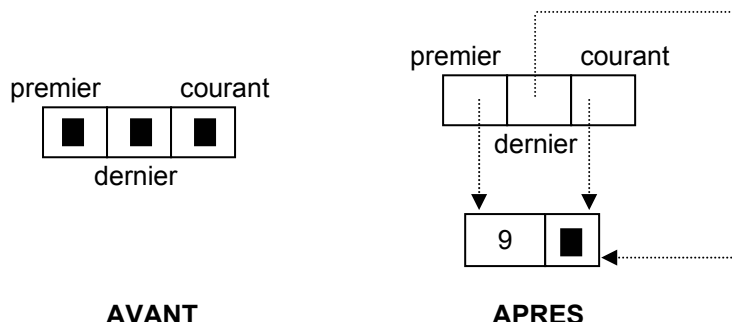
Figure IX.2 - Insertion d'un élément en position courante dans une liste vide.
