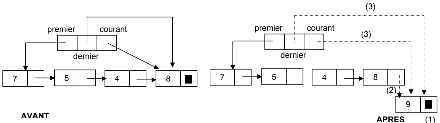
Figure IX.4 - Insertion d'un élément en dernière position dans une liste non vide.
