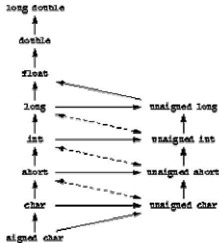
Figure II.1 - Les conversions des types en C [CL97].
