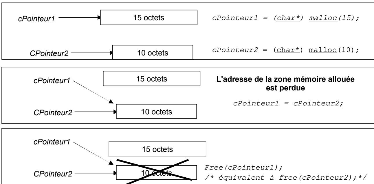
Figure II.2 - La désallocation mémoire de deux pointeurs égaux.
