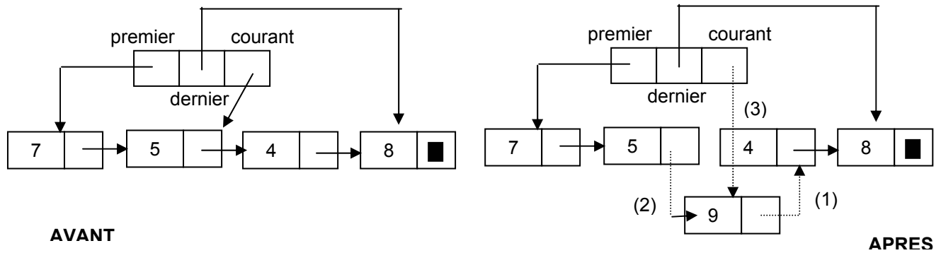
Figure IX.3 - Insertion d'un élément en position courante dans une liste non vide.
